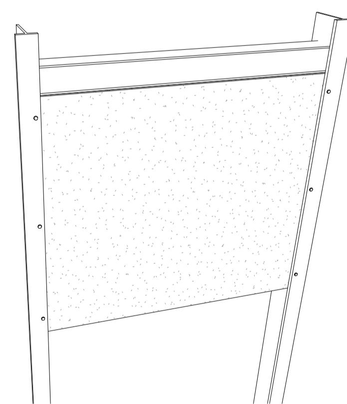
DETALHE 05 - FIXAÇÃO DO MÓDULO ESCALA: SEM ESCALA
