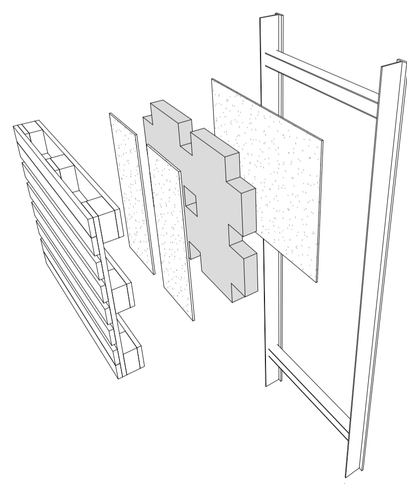
DETALHE 04 - CAMADAS ESCALA: SEM ESCALA
