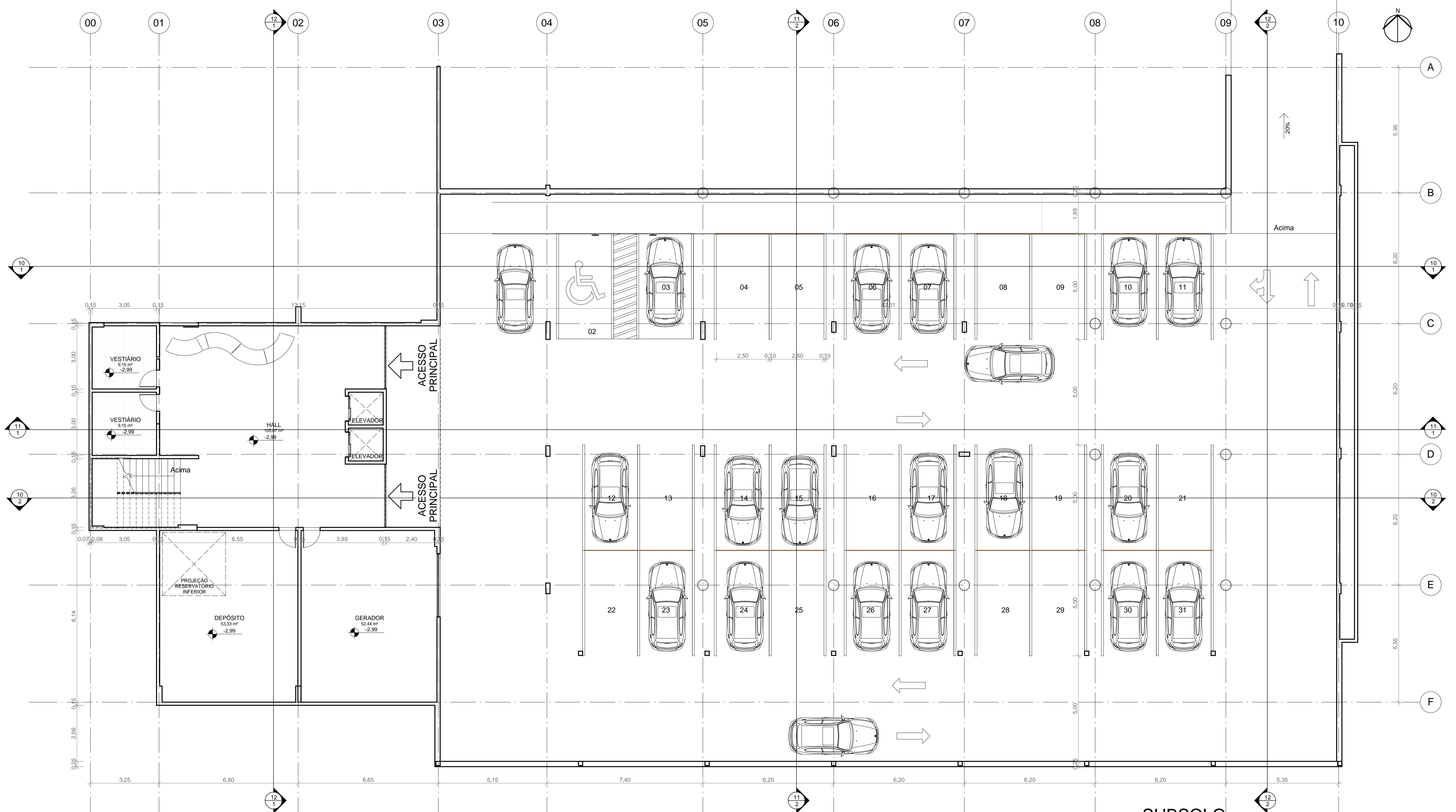
1 SUBSOLO 1 : 100
