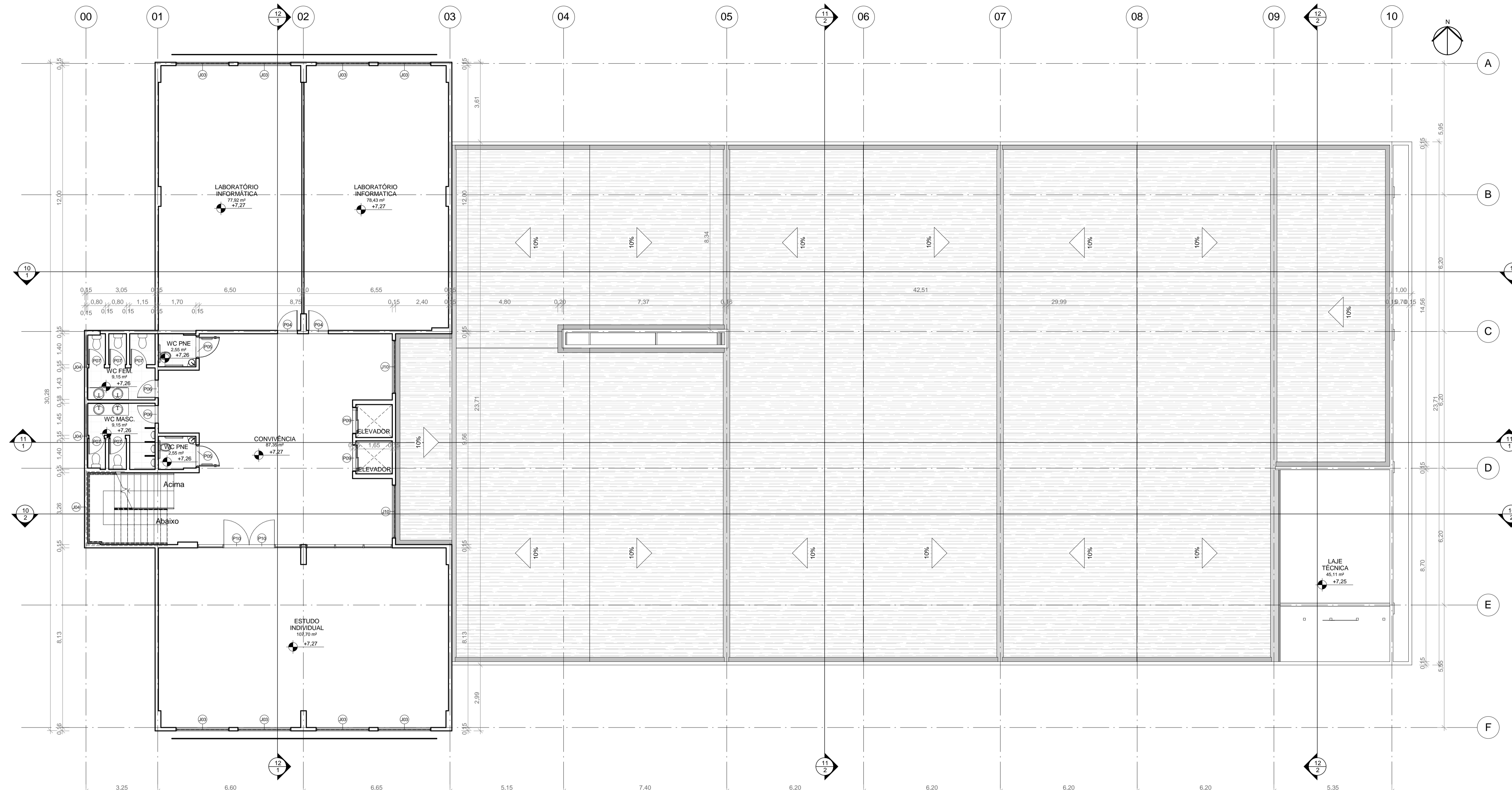
1 PLANTA BAIXA 2º PAVIMENTO 1 : 100
