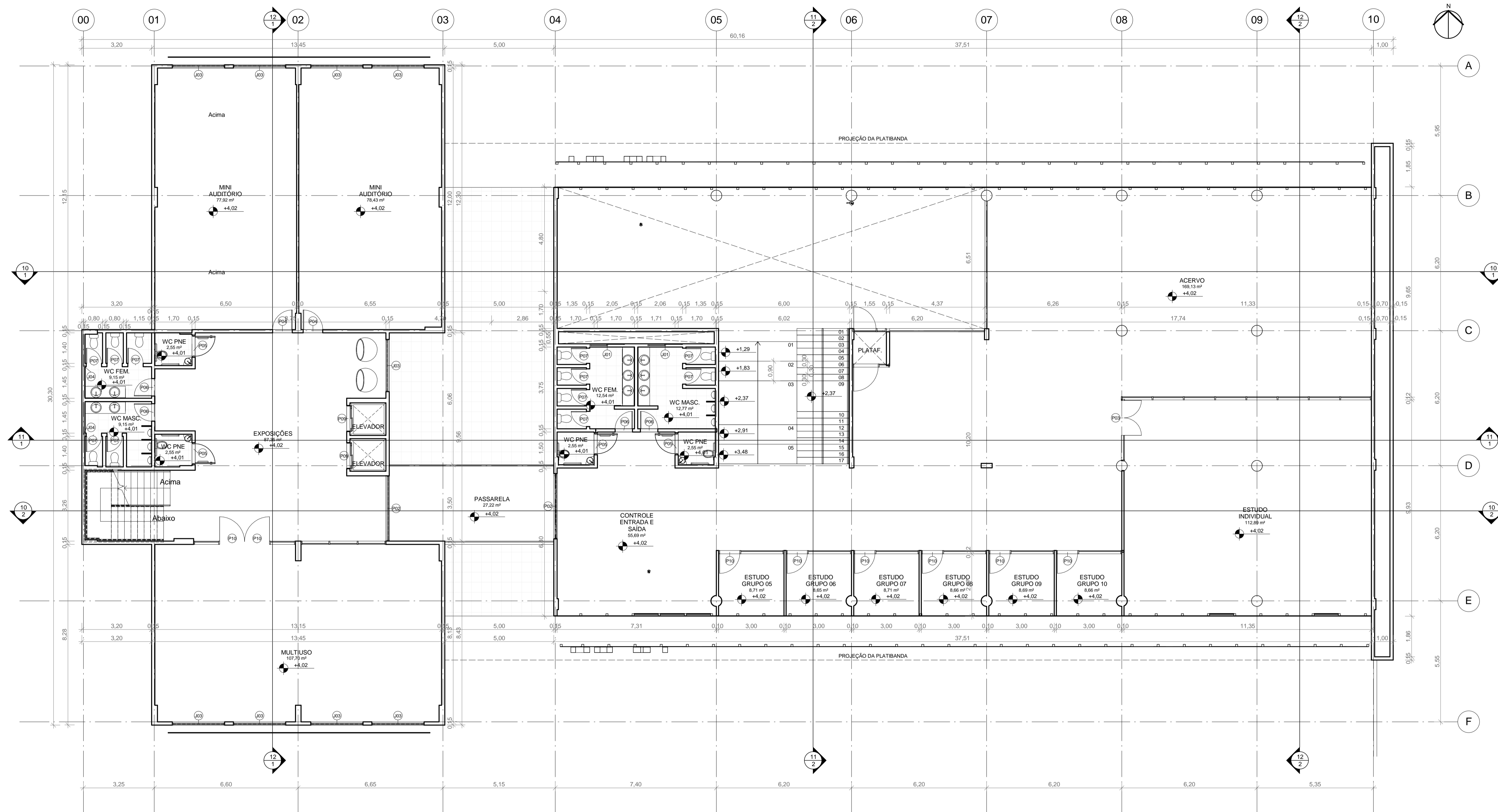
1 PLANTA BAIXA 1º PAVIMENTO 1:100
