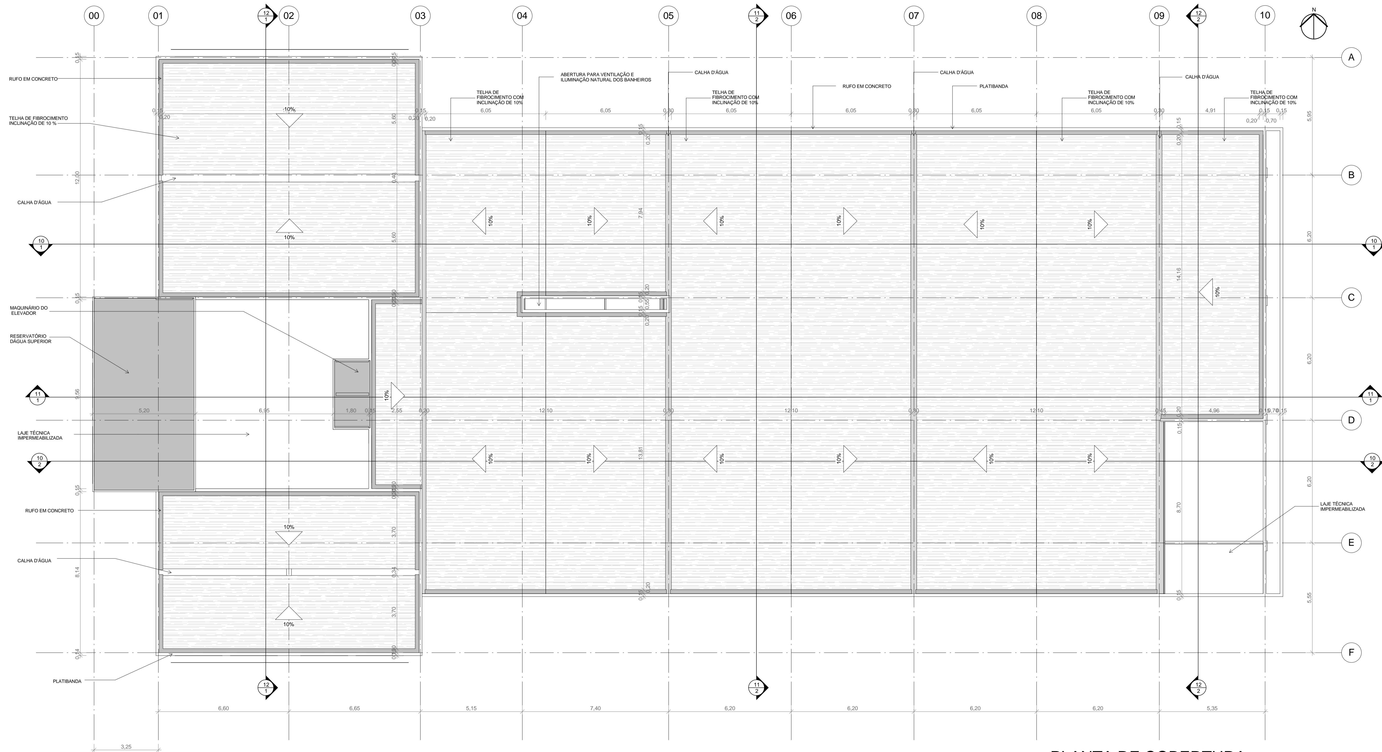
1 PLANTA DE COBERTURA 1 : 100
