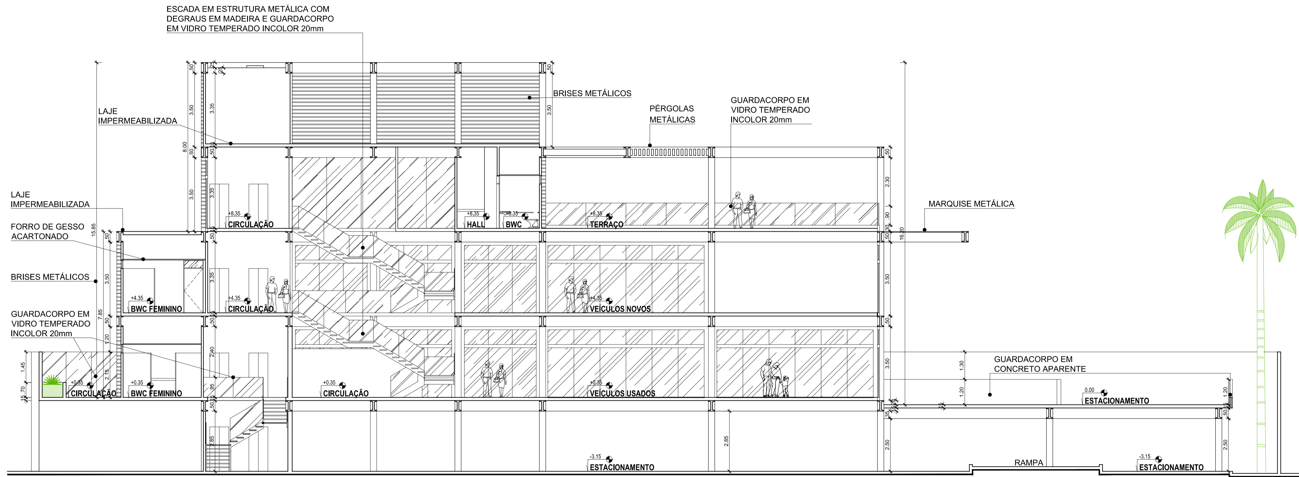
CORTE AA ESCALA 1/100
