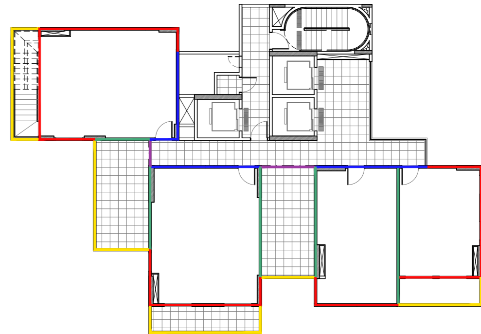
PLANTA BAIXA - PAVTO TIPO 1 (OPÇÃO A) ESTUDO DE DESEMPENHO ACÚSTICO ESCALA ..... 1/200
