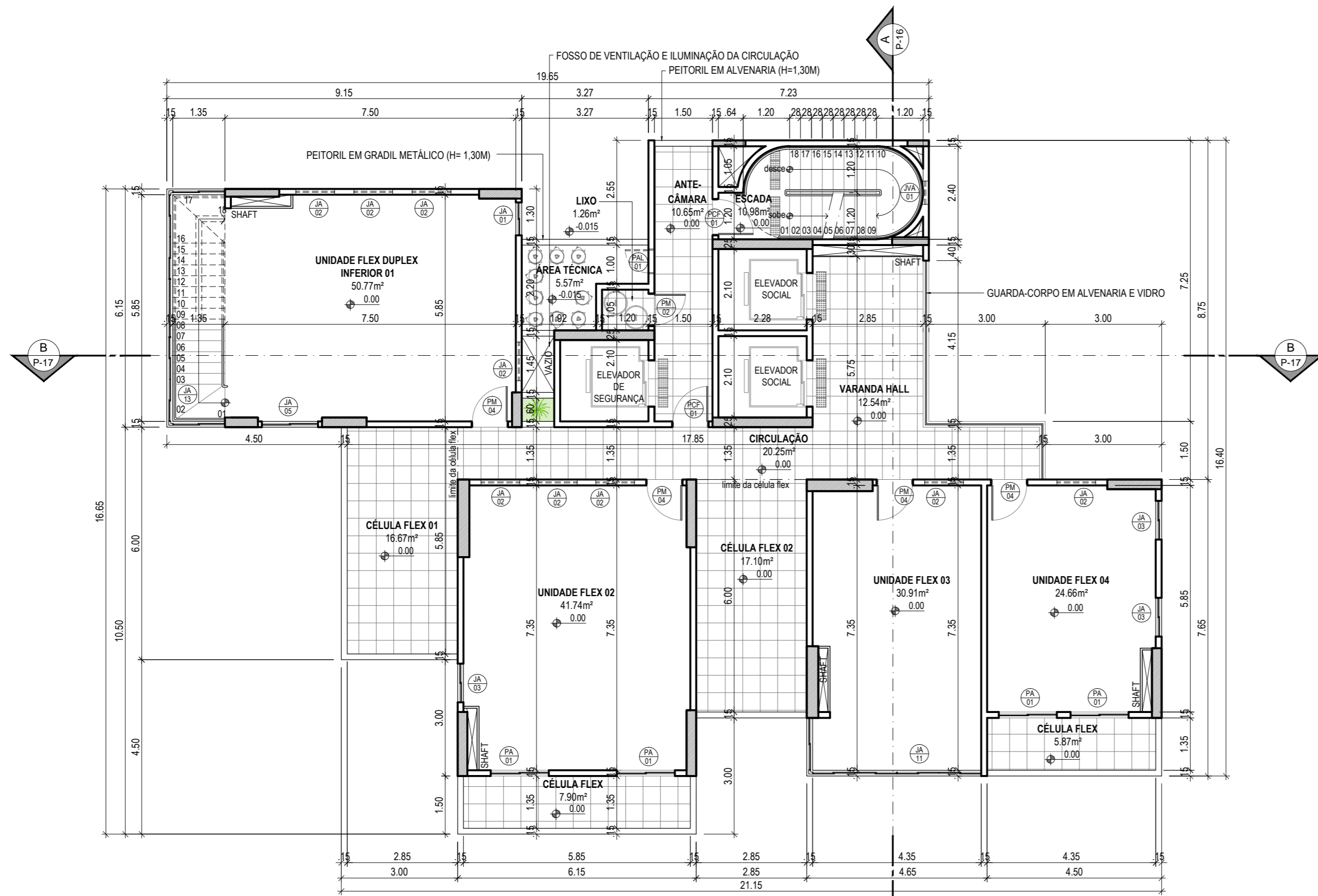
PLANTA BAIXA - PAVTO TIPO 01 (OPÇÃO A) ESCALA ..... 1/100 PAVTO TIPO DO 01 AO 18
