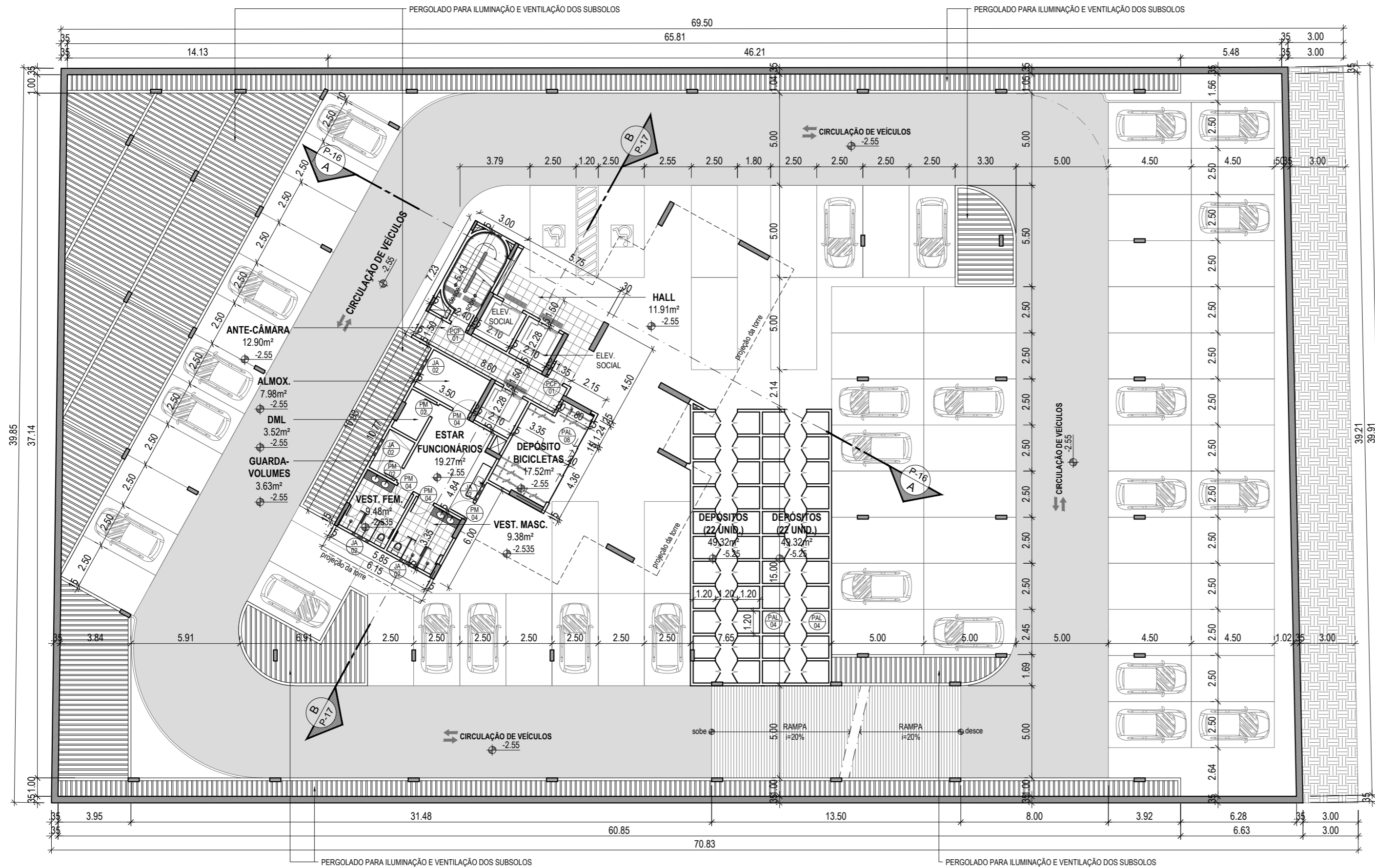
PLANTA BAIXA - PAVTO SUBSOLO 01 ESCALA ..... 1/200
