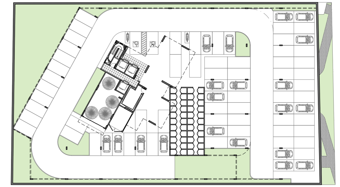
PLANTA BAIXA - PERMEABILIDADE ESCALA ..... 1/500 LEGENDA PERMEABILIDADE 100% (JARDIM OU COBOGRAMA) PERMEABILIDADE 50% (PISO INTERTRAVADO) PERMEABILIDADE 0% (LAJE)
