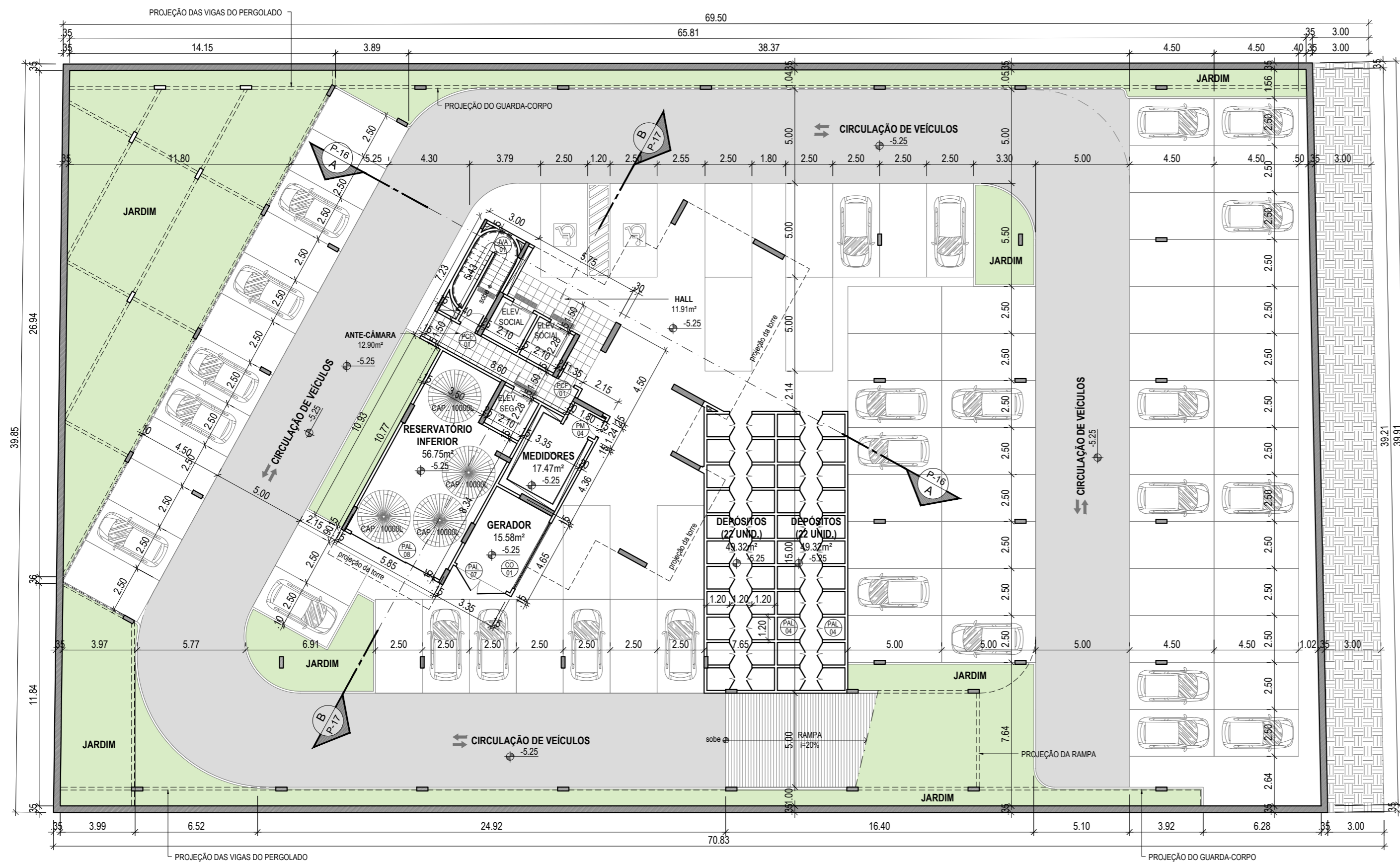
PLANTA BAIXA - PAVTO SUBSOLO 02 ESCALA ..... 1/200
