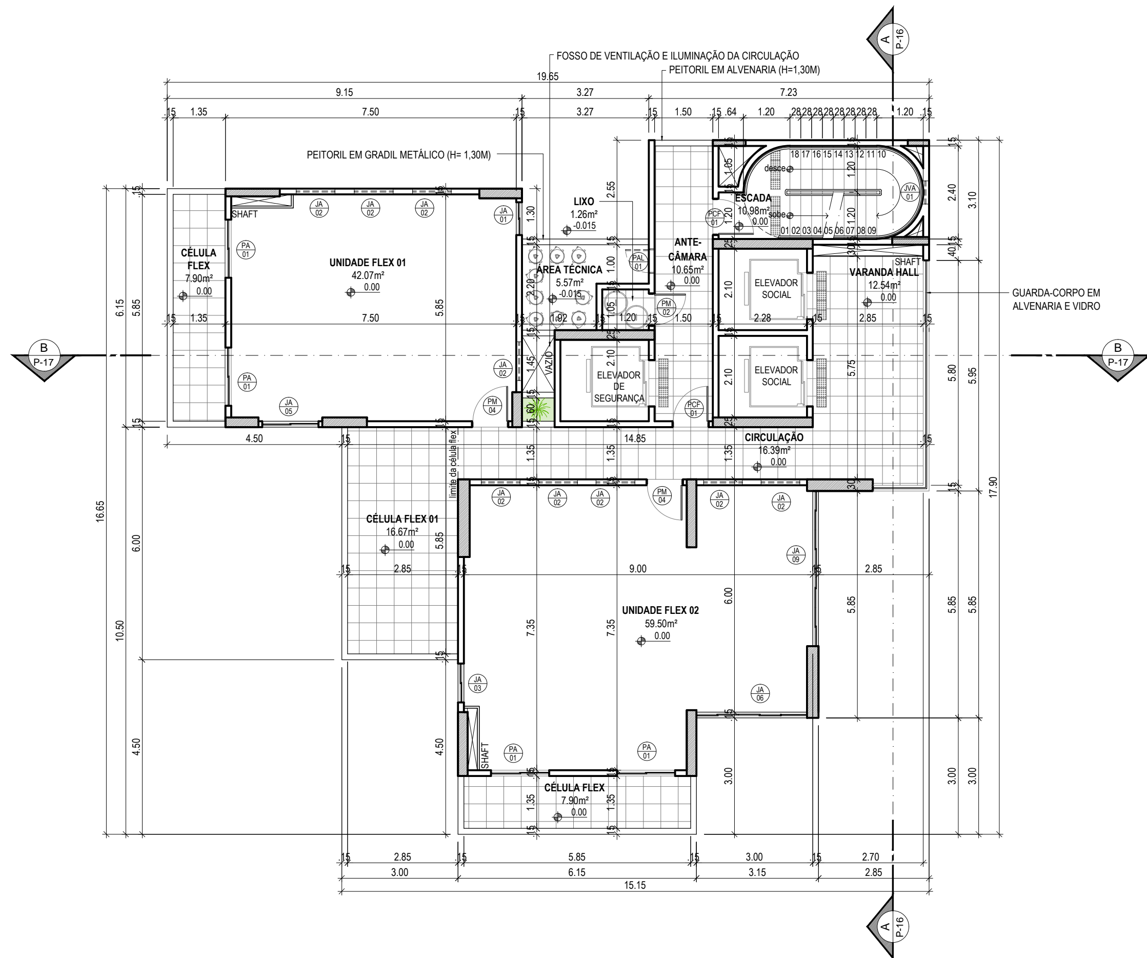
PLANTA BAIXA - PAVTO TIPO 03 (OPÇÃO B) ESCALA ..... 1/75 PAVTO TIPO DO 20 AO 23
