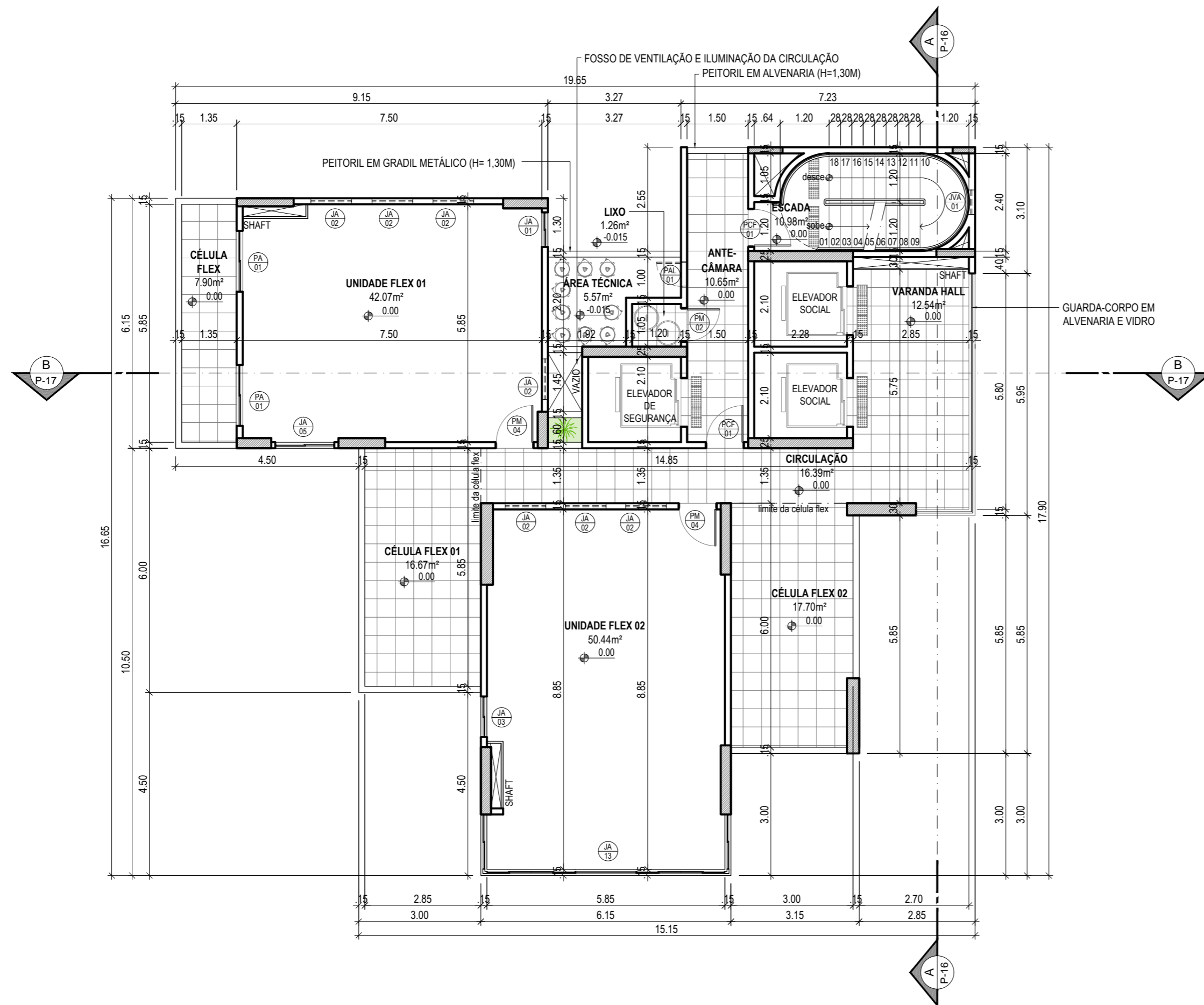
PLANTA BAIXA - PAVTO TIPO 03 (OPÇÃO A) ESCALA ..... 1/100 PAVTO TIPO DO 20 AO 23
