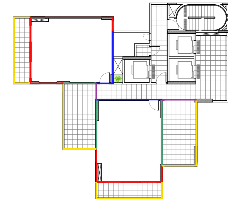
PLANTA BAIXA - PAVTO TIPO 3 (OPÇÃO A) ESTUDO DE DESEMPENHO ACÚSTICO ESCALA ..... 1/200
