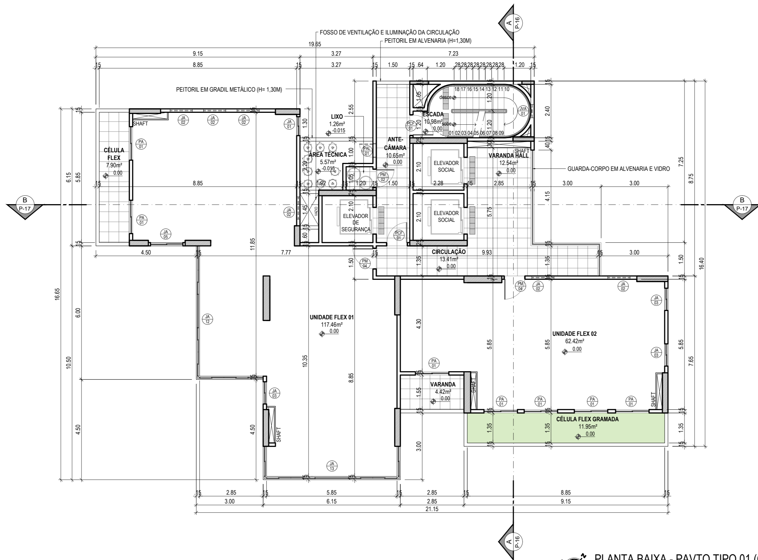
PLANTA BAIXA - PAVTO TIPO 01 (OPÇÃO C) ESCALA ..... 1/100 PAVTO TIPO DO 01 AO 18
