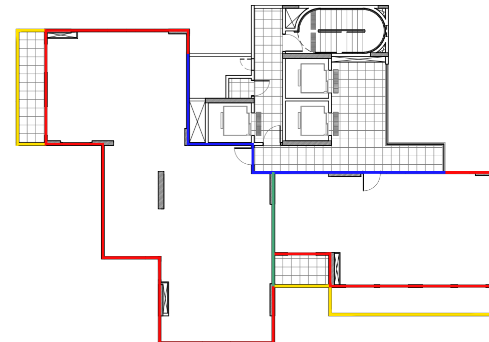
PLANTA BAIXA - PAVTO TIPO 1 (OPÇÃO C) ESTUDO DE DESEMPENHO ACÚSTICO ESCALA ..... 1/200
