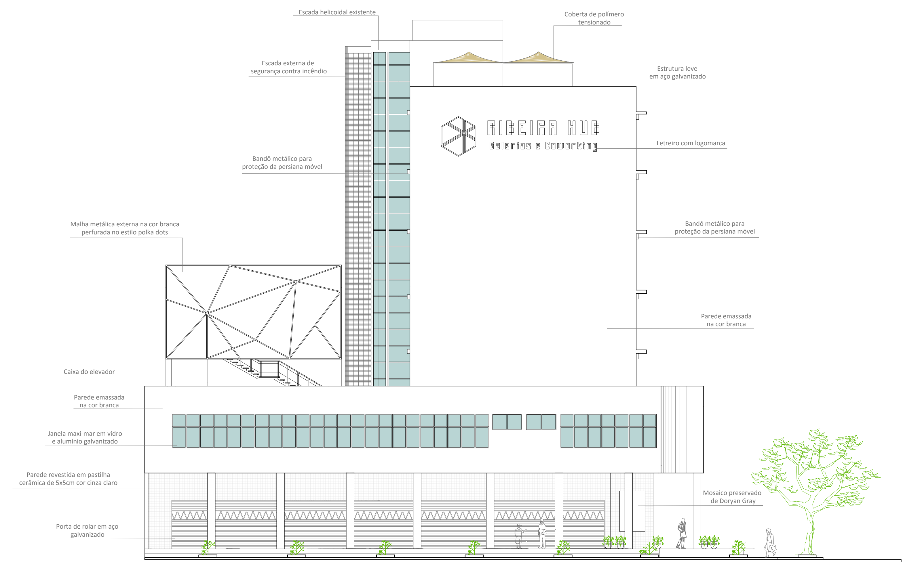
FACHADA SUL ESCALA.....1/125
