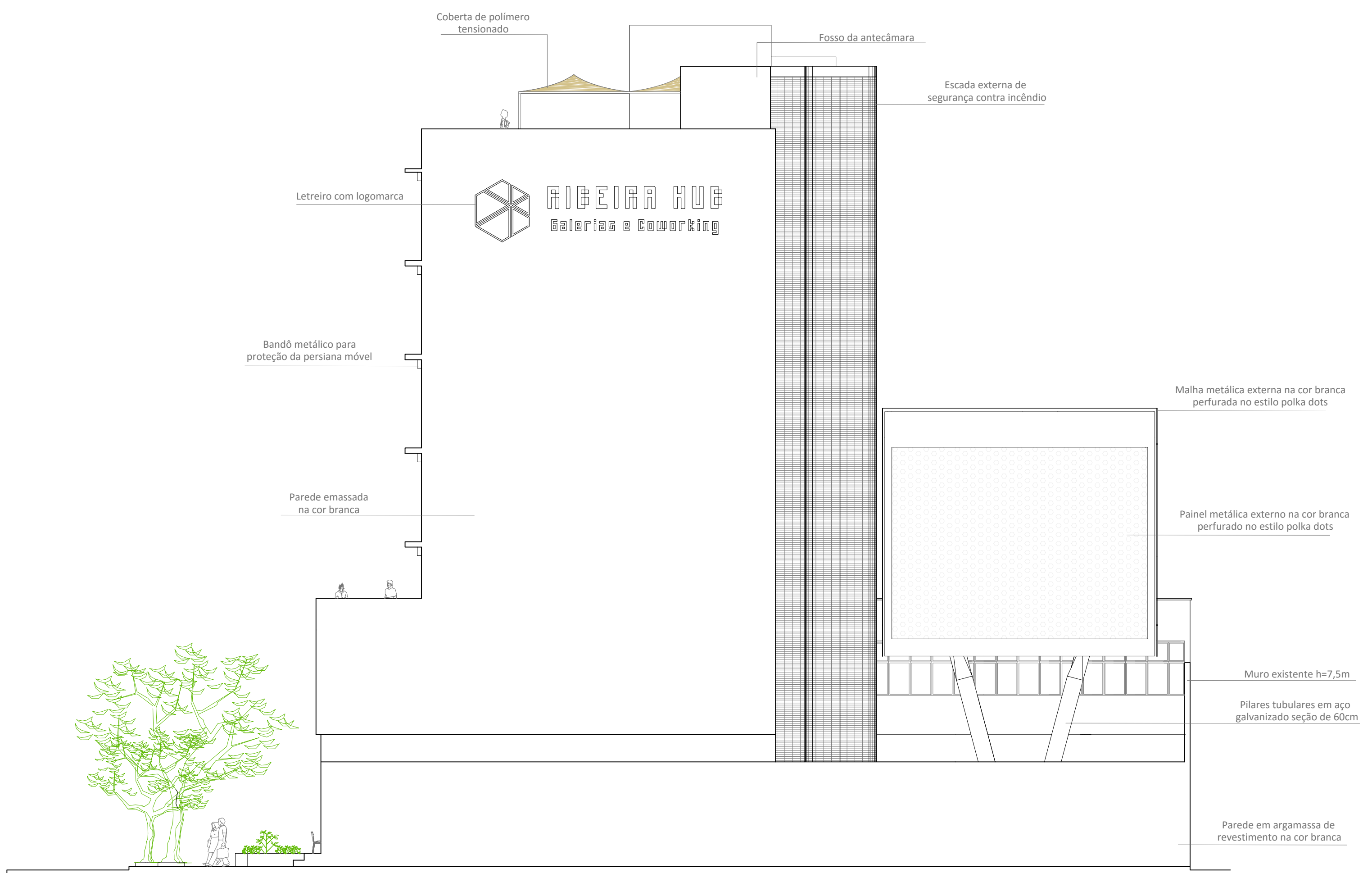
FACHADA NORTE ESCALA.....1/125
