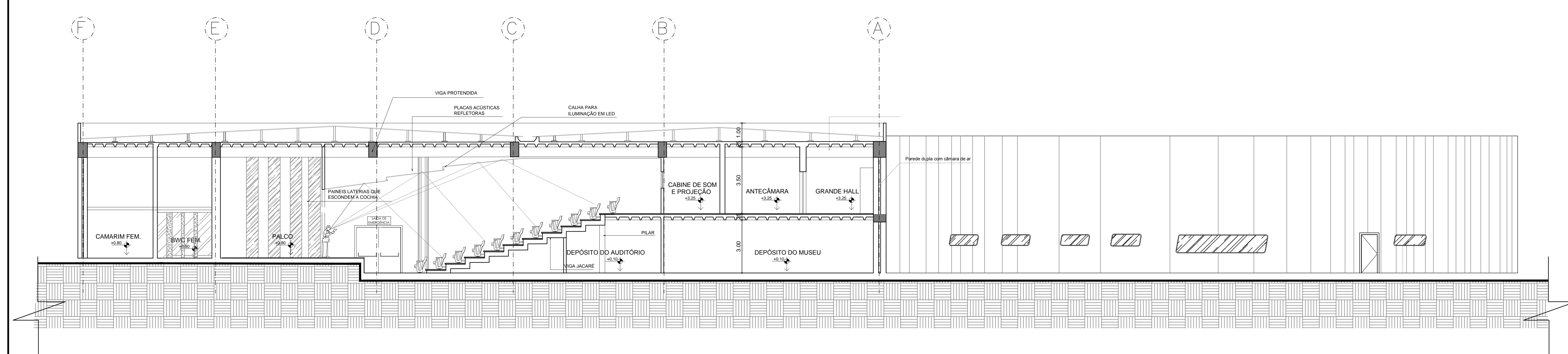
CORTE BB ESCALA 1/100
