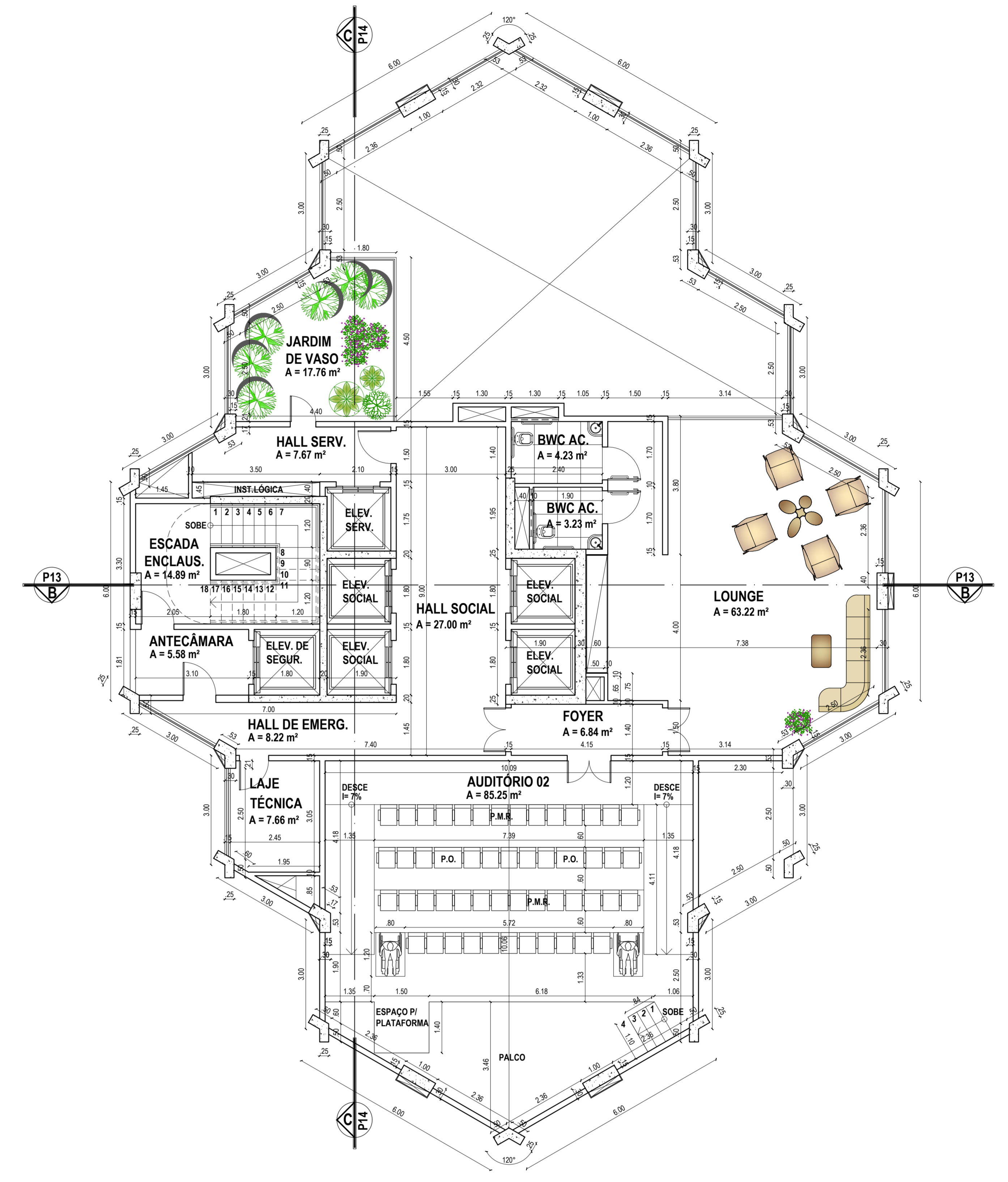
PLANTA BAIXA - PAV. DE MEZANINO DO EDIFÍCIO 02 ESCALA ..... 1/75
