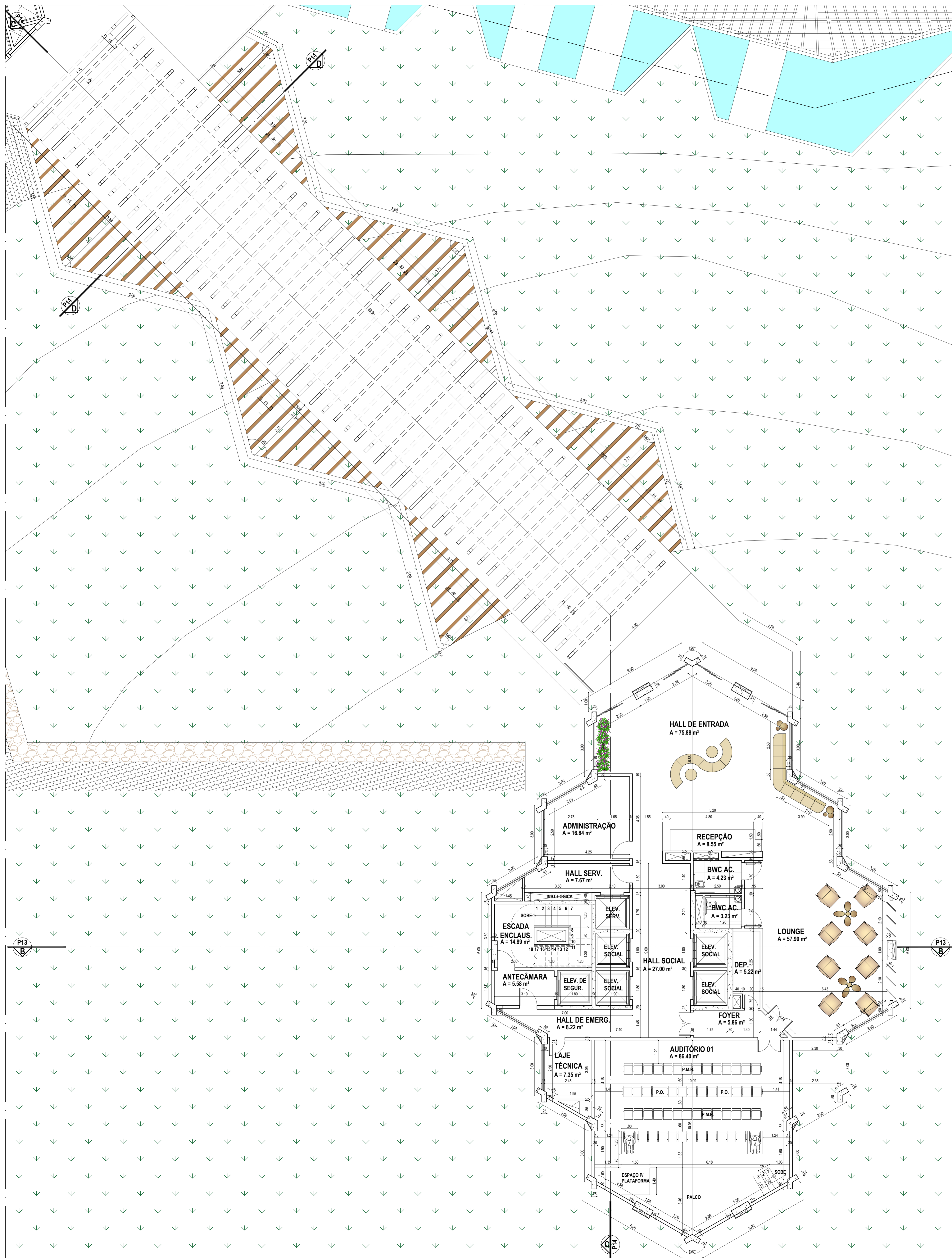
PLANTA BAIXA - PAV. DE RECEPÇÃO DO EDIFÍCIO 02 E PASSARELA ESCALA ..... 1/75
